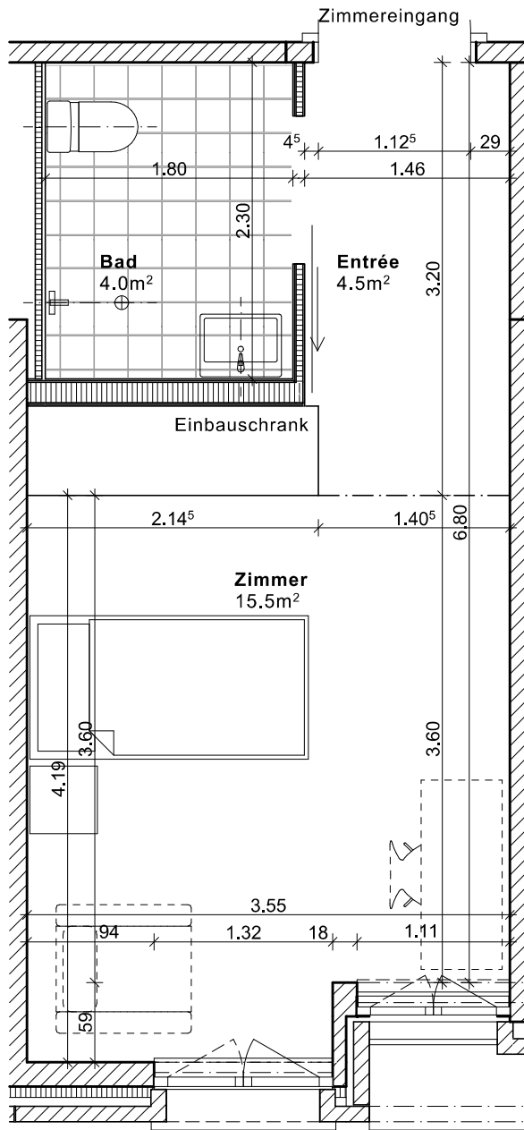
Grundriss, 1:50
