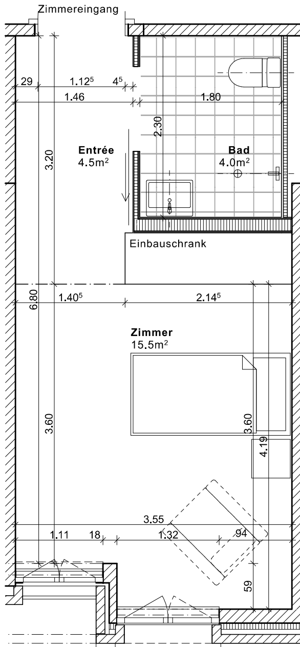
Grundriss, 1:50
